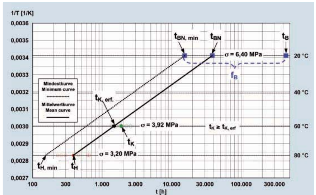
Bild 3: Prüfbedingungen nach dem MAC-Konzept für HS-Schweißverbindungen aus PE 80 [4]
