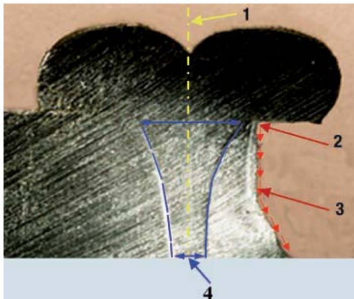
Bild 2: Vereinfachte Methode zum Mindestnachweis eines geforderten Zeitstandzug-Schweißfaktors, Bild 6 aus [1]
